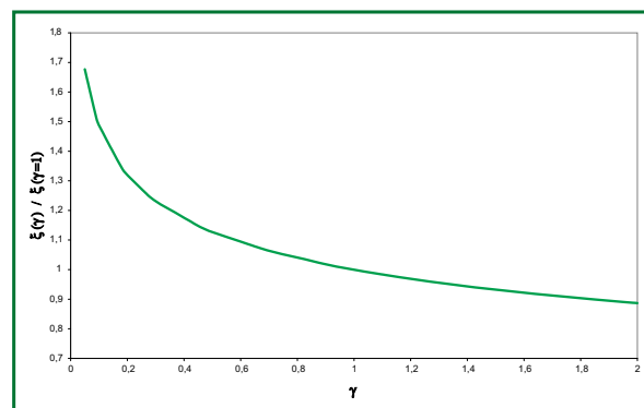
Variazione media del coefficiente di smorzamento viscoso equivalente \xi in funzione della deformazione di taglio \gamma .
