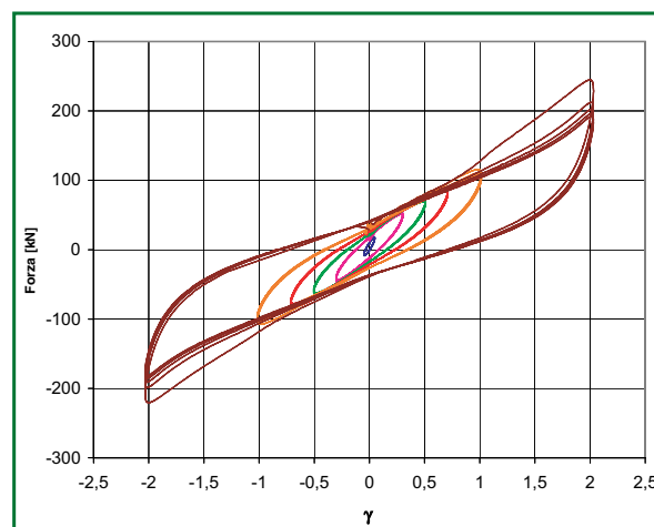
Tipico diagramma isteretico di un isolatore elastomerico ottenuto in prove dinamiche ad ampiezza crescente.
